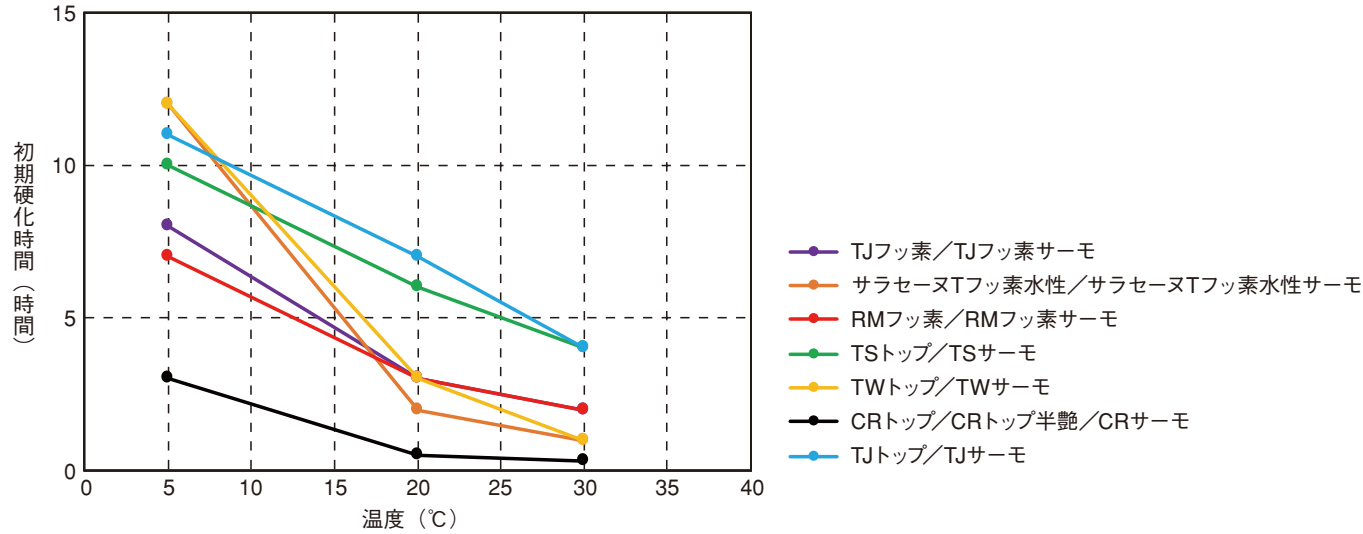
初期硬化時間の目安
