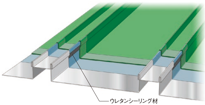
瓦棒屋根MR工法
