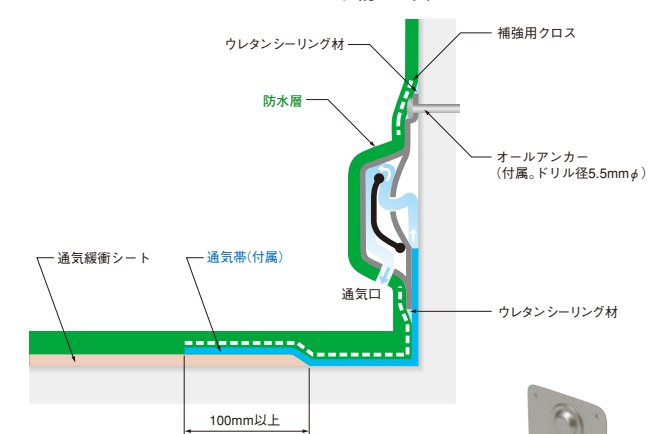
SR パラベント納まり図
